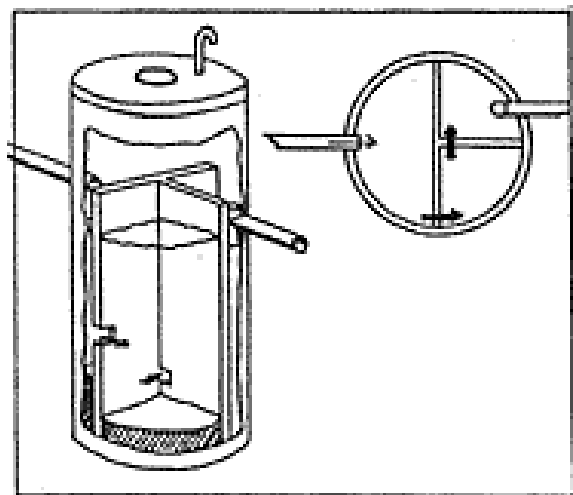
Bild: Slamavskiljare (genomskärning och från ovan)
